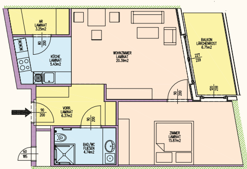
Musterplanung Wohnung Generationenhaus
